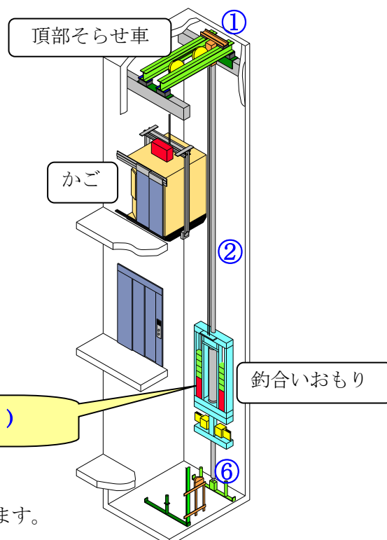
リニア式の検査項目と検査箇所の外観図
